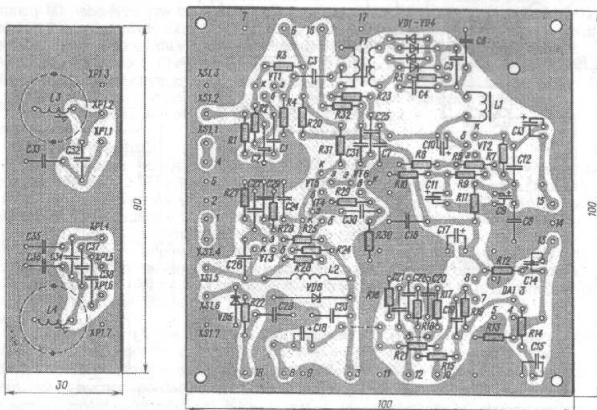
обр. 4 Проведение плоских spojů a osazení součástkami
