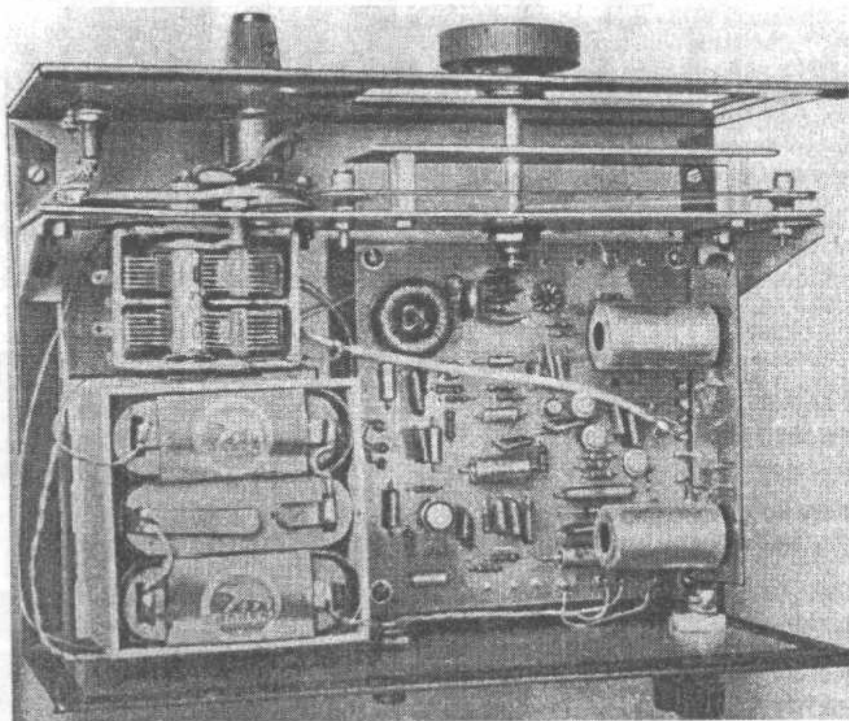
obr. 8 Vnitřní uspořádání přijímače.
