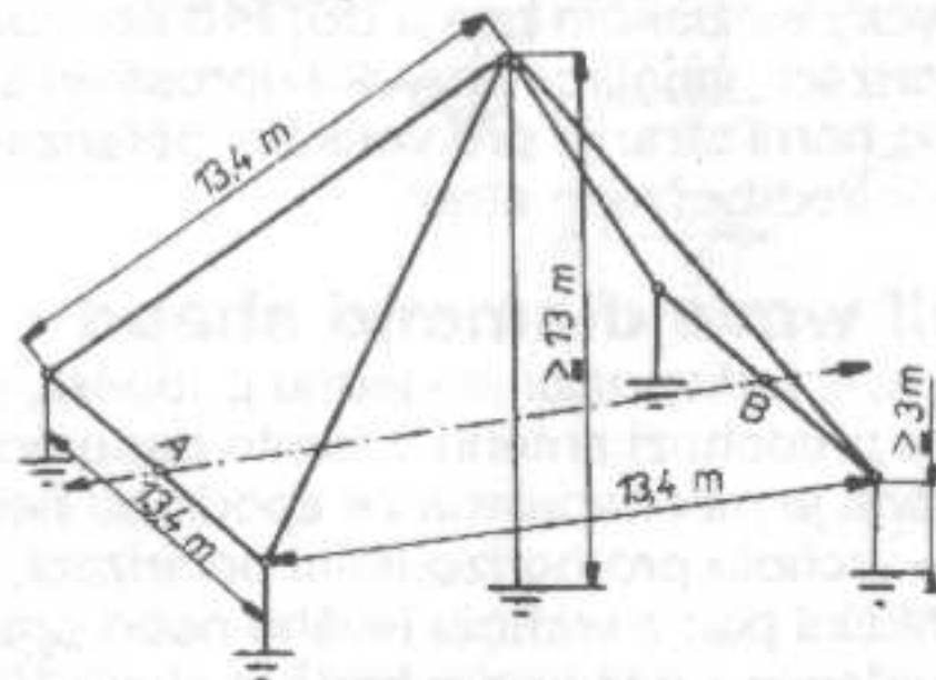
Provedení a rozměry antény pro pásmo 80 m
