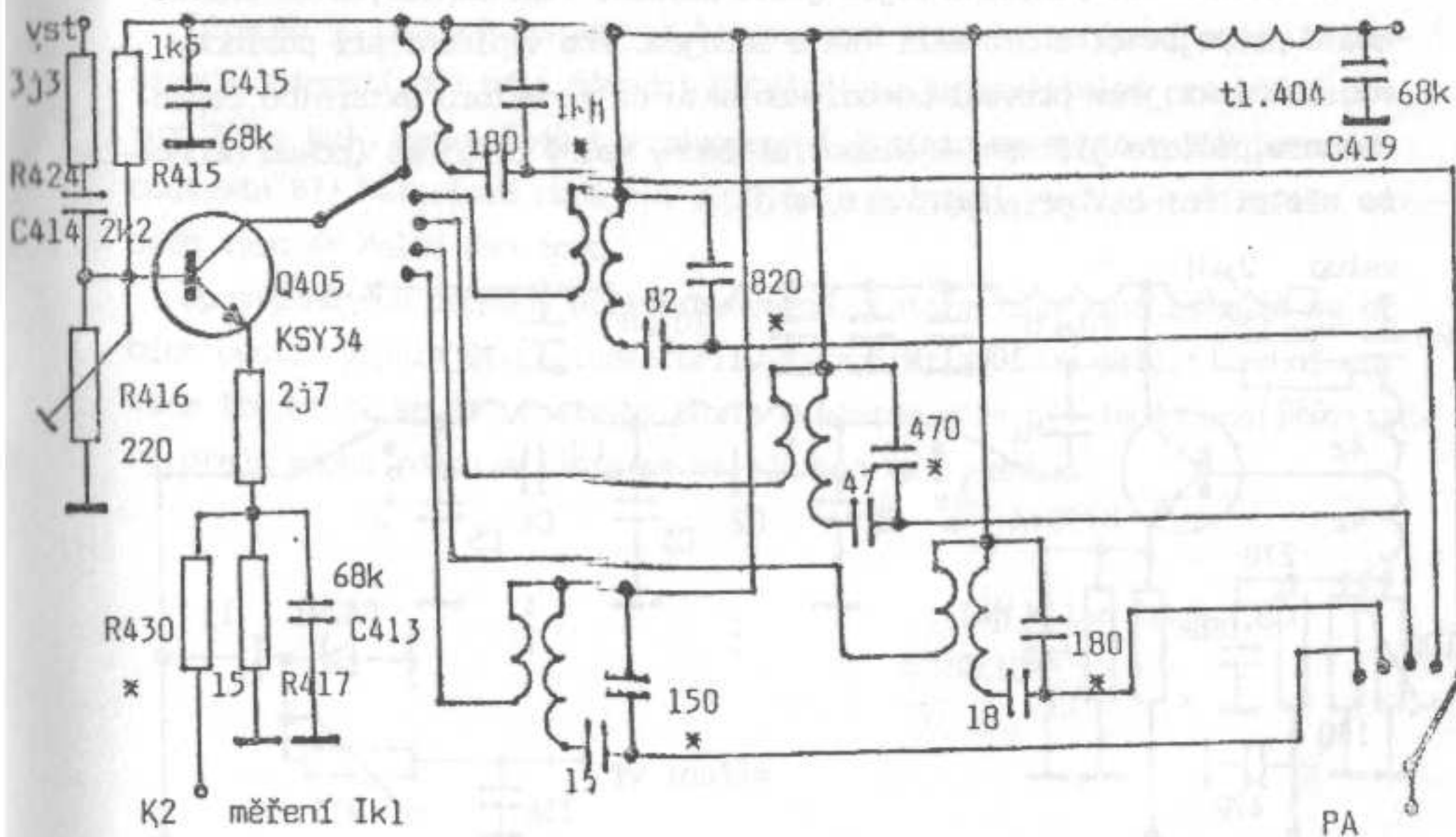
Obr.6. Budič PA.
