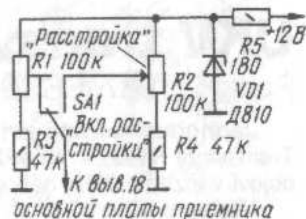
obr. 10 Obvod RITu
