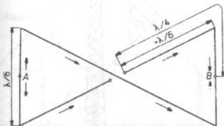
Orientace proudu v anténě
