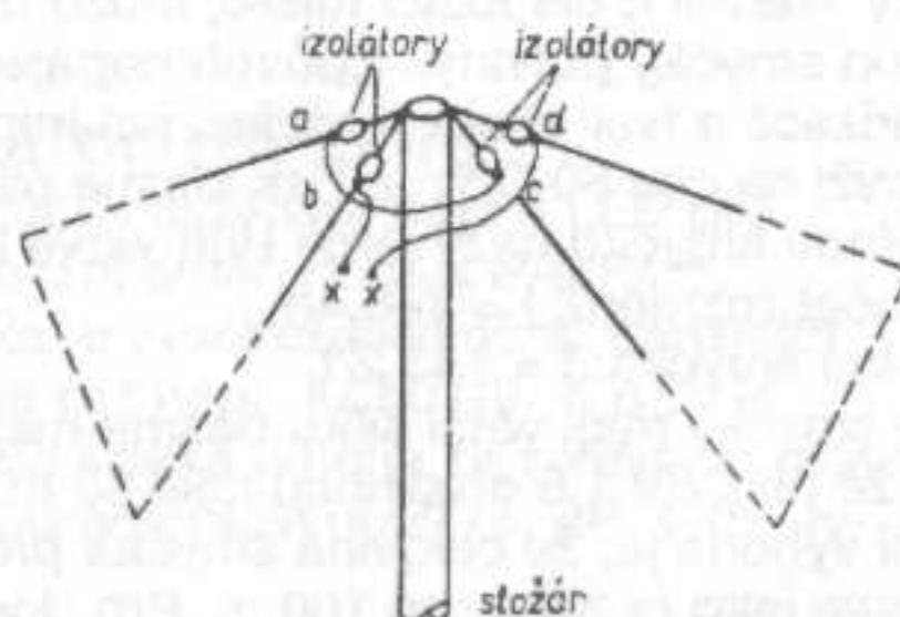
Detail upevnění izolátorů
