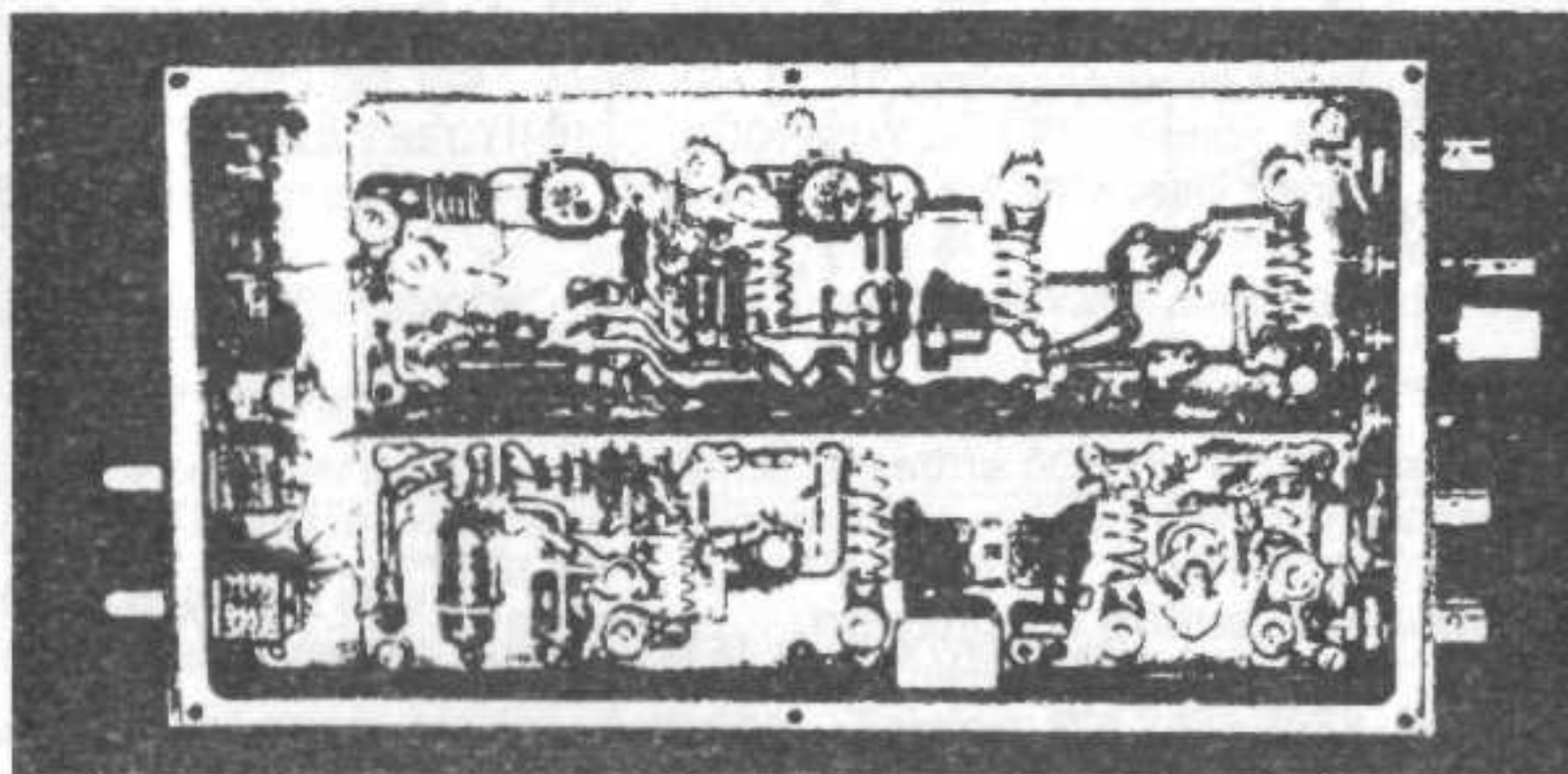
obr. 4 pohled na osazenou desku plošných spojů
