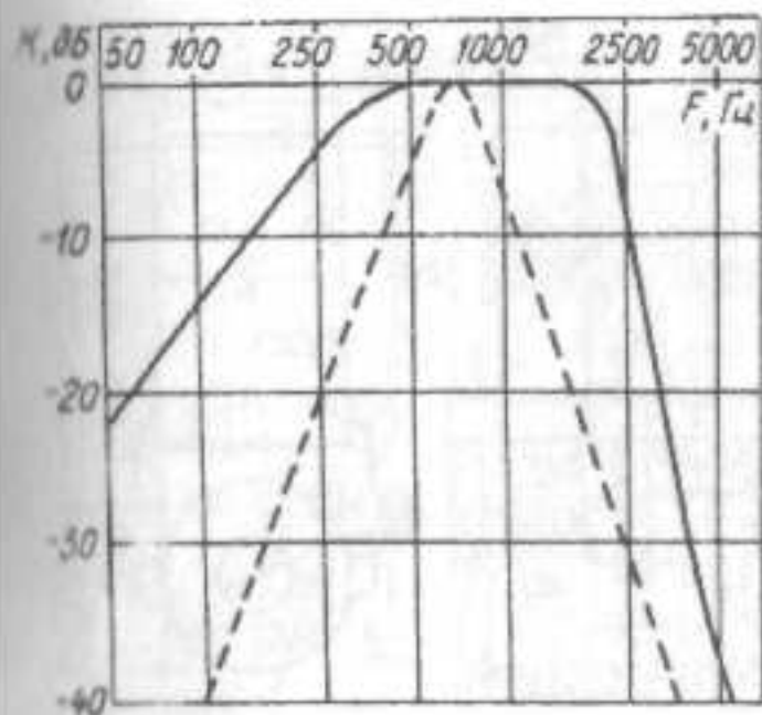
obr. 6 Průběh kmitoč- tové charakteristiky pro CW a SSB
