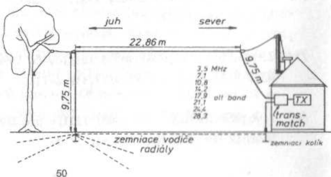
Obr. 5. Grounded half-loop. Celková délka 42,36 m
