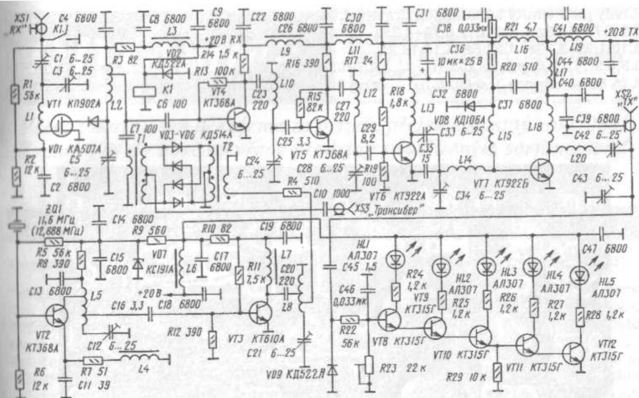
obr. 1 schéma zapojení
