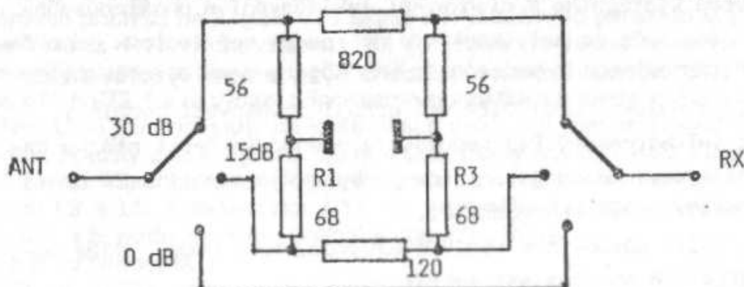
Obr. 1. Atenuátor RX
