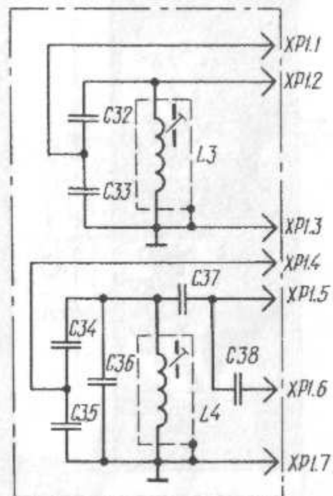
obr. 3 Zapojení výměnných cívkových sad
