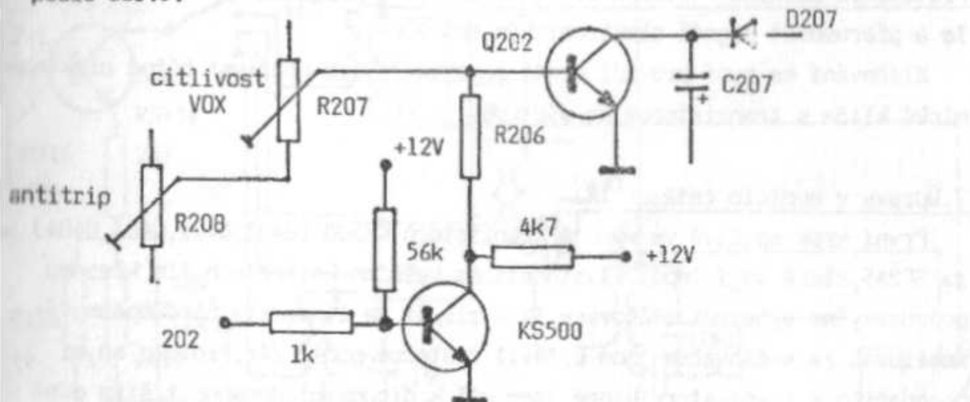
Obr.3. Úprava VOX.
