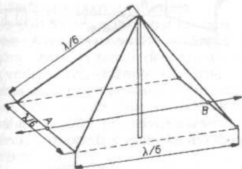
Náčrt antény
