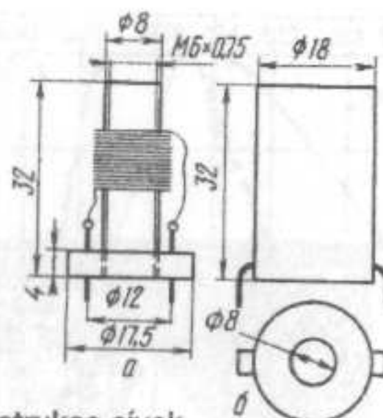
Obr. 9 Konstrukce cívek
