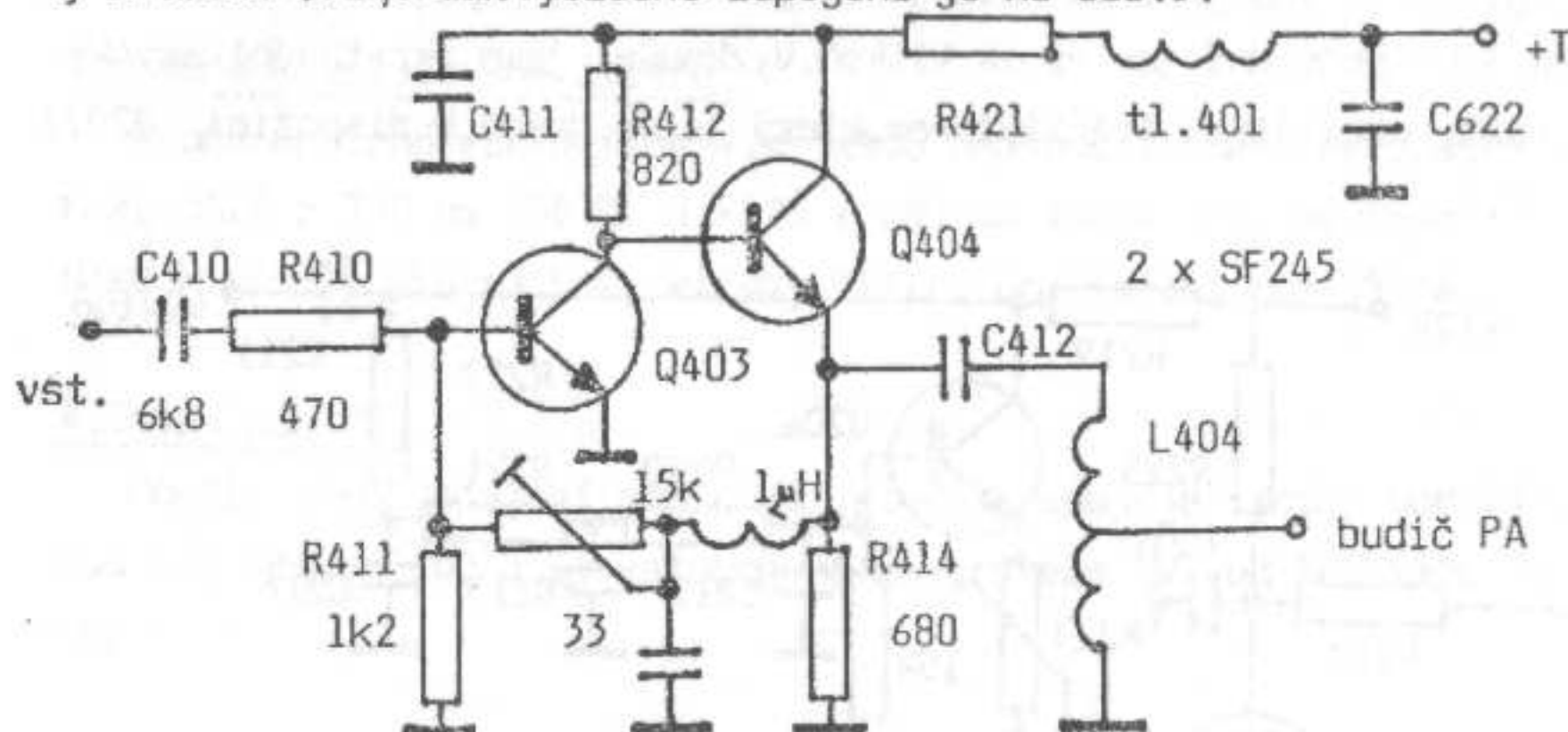
Obr. 5. Širokopásmový zesilovač budiče.
